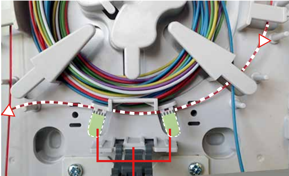
Guide-câble avec pattes de guidage sécables Cable guide with breakable legs
