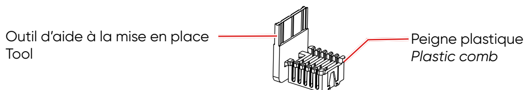
Fig. Peigne pour micromodule Ø900 µm et outil d'aide à la mise en place Plastic comb for Ø900 µm microbundle and its tool
