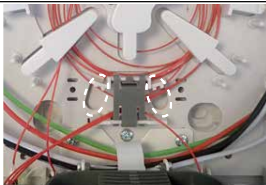
Fig. Passage de câbles en configuration loosetube Cable routing - loosetube configuration
