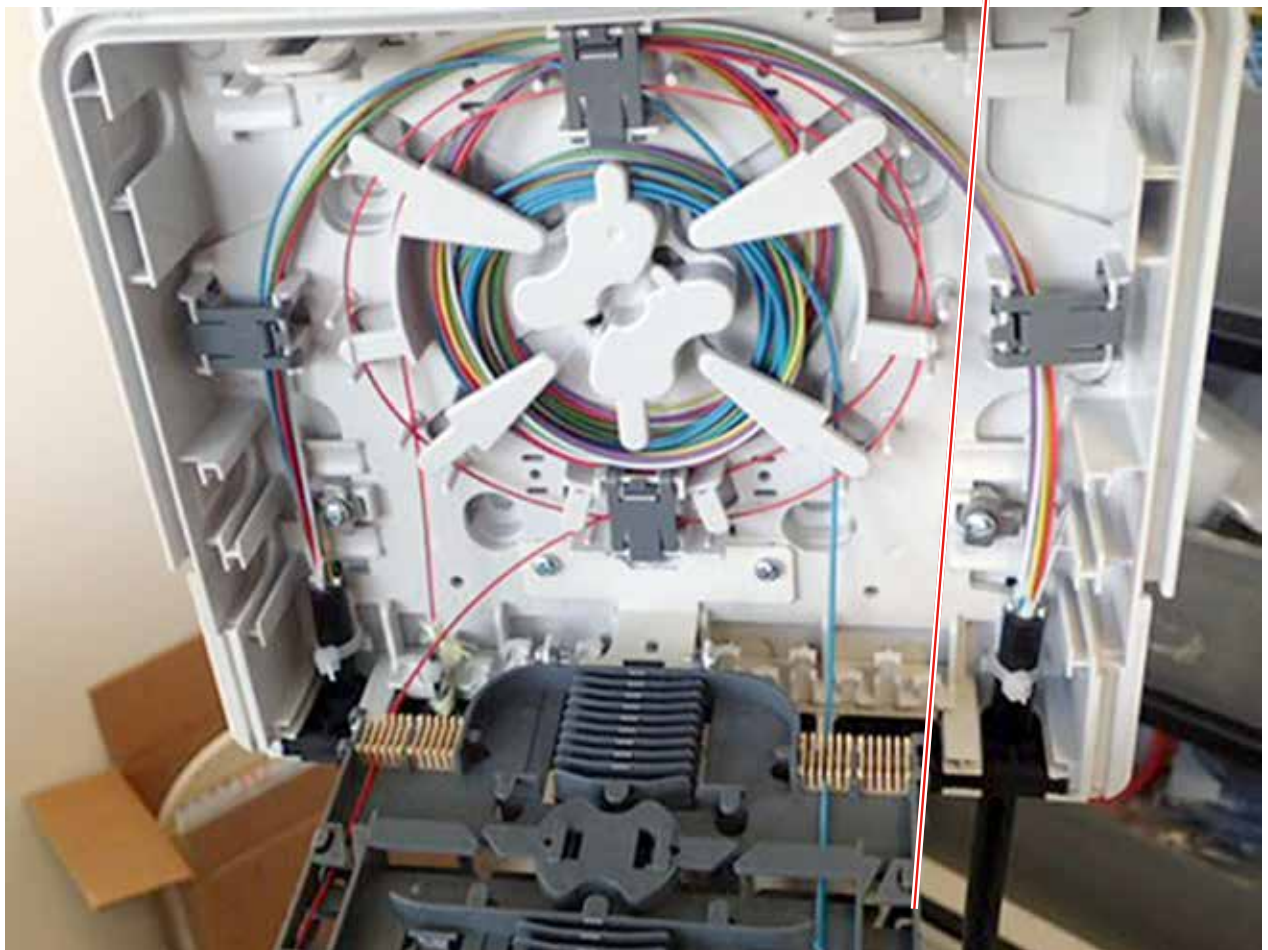
Fig. Cheminement des fibres à dériver - Vue face intérieure cassette Routing of fibres to be shunted - Tray inner side view
