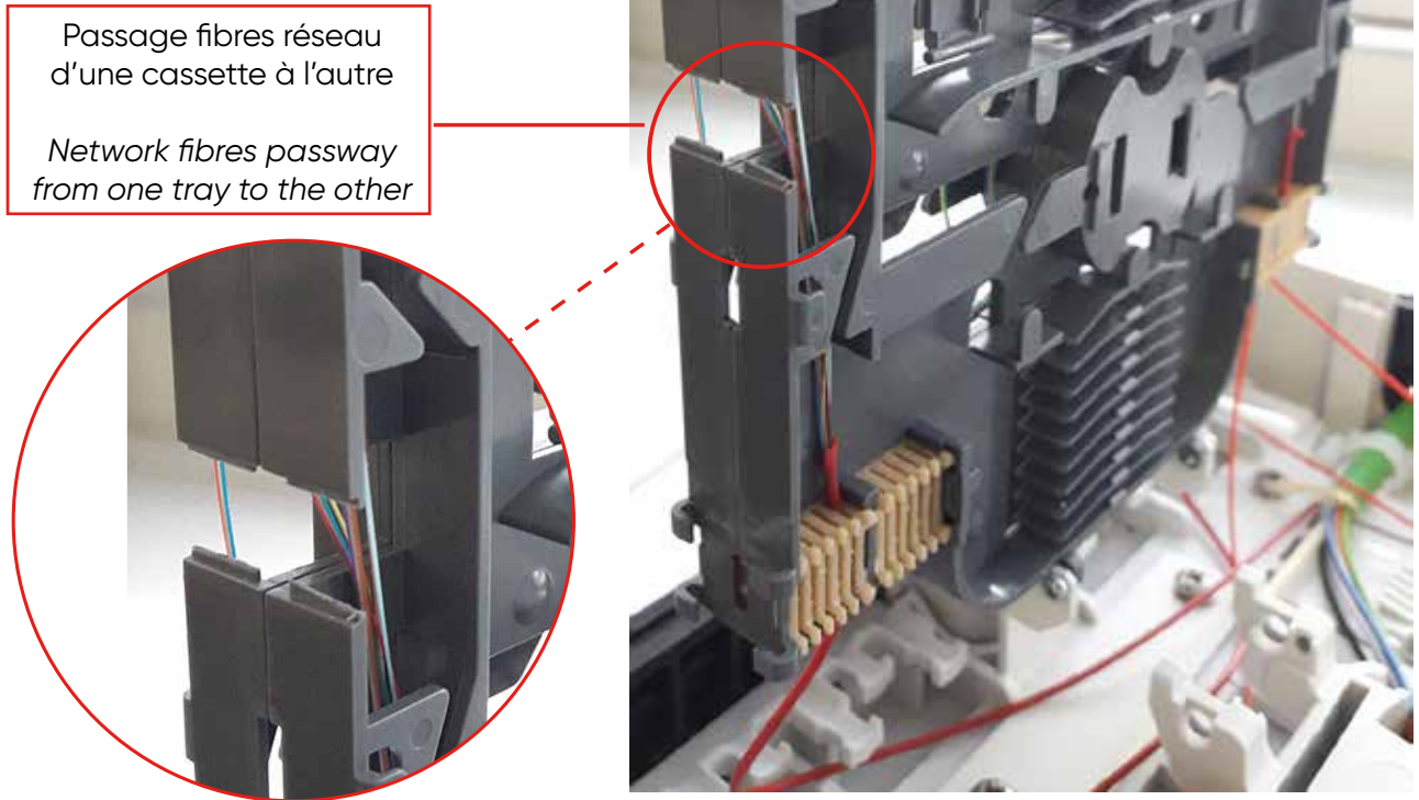
Fig. Utilisation du bord sécable de la cassette d'épissurage Using the removable edge of the splicing tray
